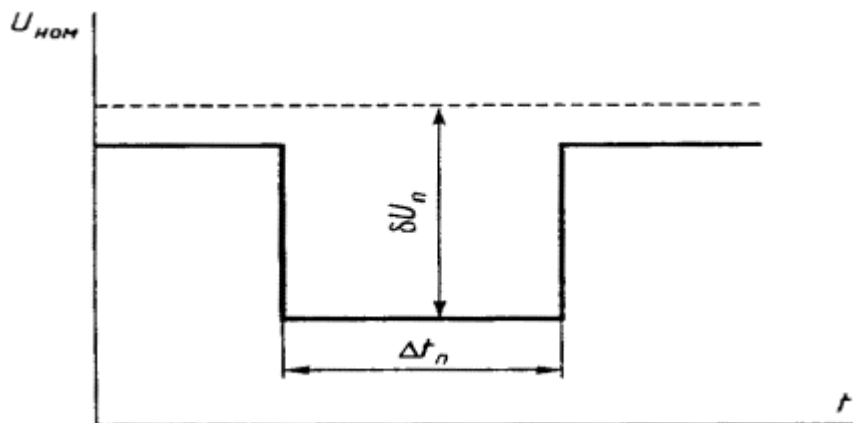
Рисунок Б.2 - Провал напряжения
